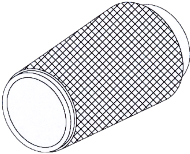
02-184cu Upper roller 上滾花鋼輪 外圓直徑 Inner Diameter 42mm & 47mm
